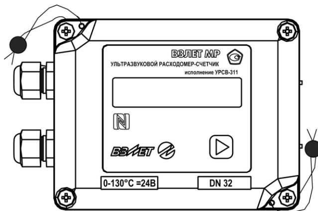
Рис.33. Внешние пломбы.
