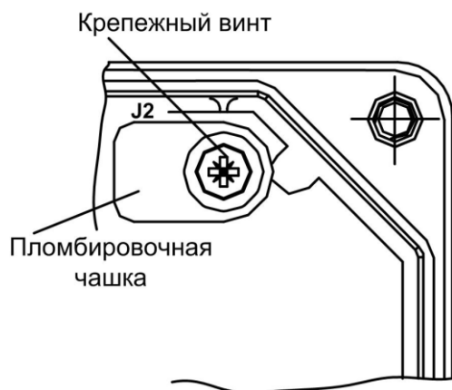
Рис.32. Пломбирование контактной пары J2.
