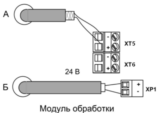
Рис.5а. Только универсальный выход при внешнем питании.
